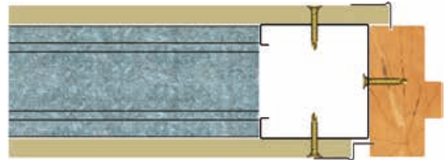
典型细节-木门框固定在DUPLEX Stud®立骨并使用阴影角线
