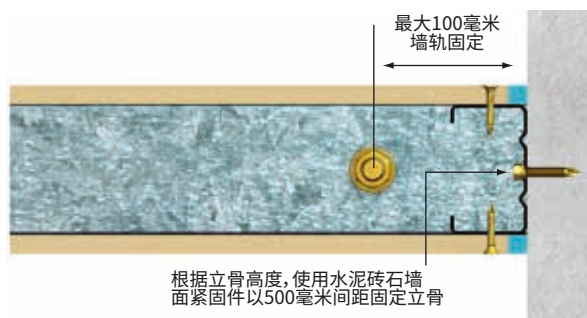
图1: 交接处 - 水泥砖石墙面
