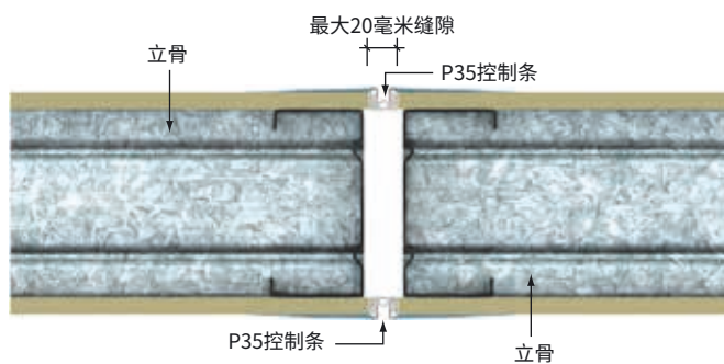
图3: 安装控制条的立骨墙体结构
